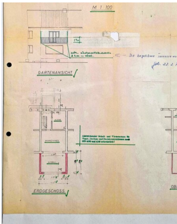
Zeichnung EG
